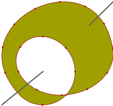
eofill
