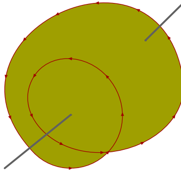
fill
